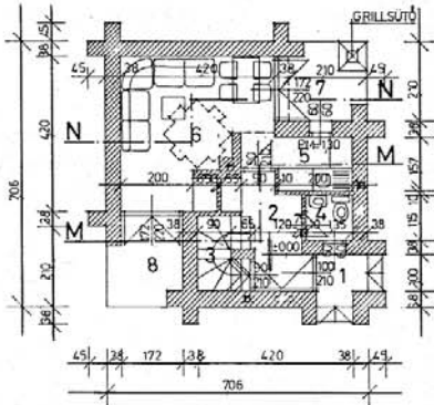
FÖLDSZINT ALAPRAJZA
