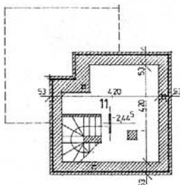
PINCESZINT ALAPRAJZA
