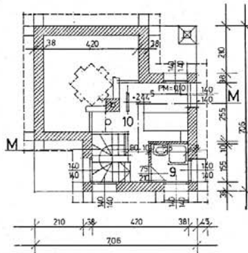
GALÉRIASZINT ALAPRAJZA
