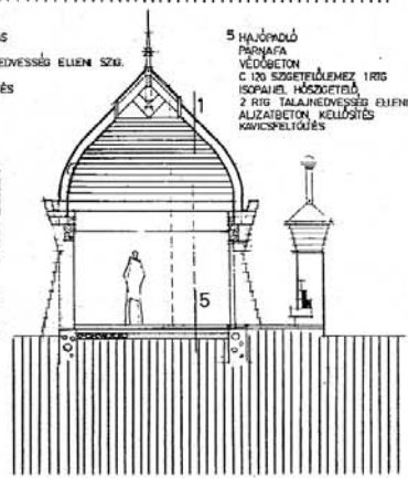
N-N METSZET
