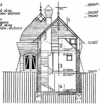
M-M METSZET
