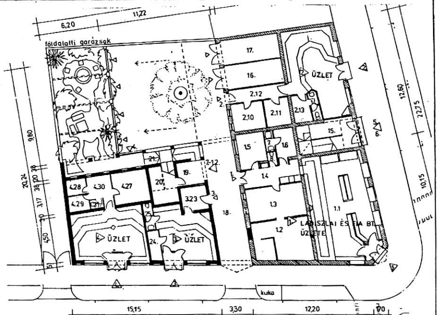
Földszinti alaprajz m 1:200 4216 m 2
