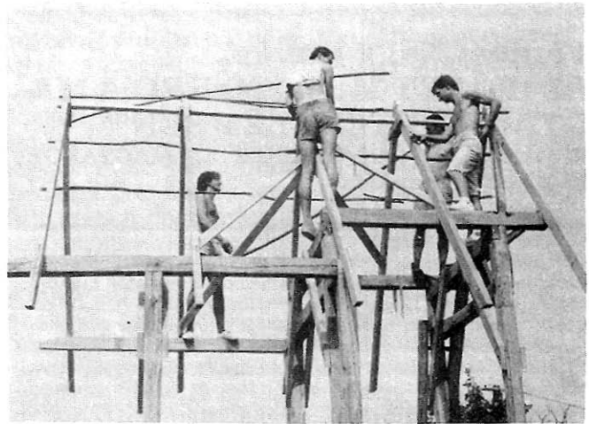
Készül a kuglizó fedélszéke
