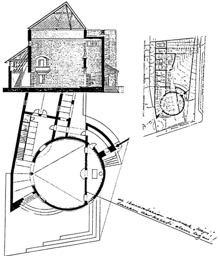
A kazincbarcikai g. templom T. alk. Főterv, 1988.02.
