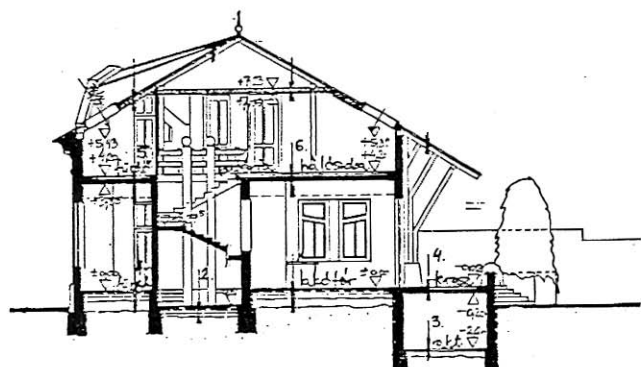
lakóház átalakítás-bővítés Kaposvár 1991-92
