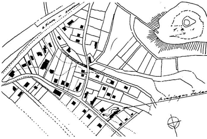
Ábrahámhegy, római katolikus templom helyszínrajza és keleti nézete
