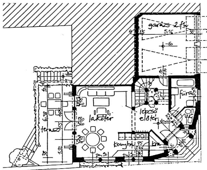
lakóház átalakítás-bővítés Kaposvár 1991-92
