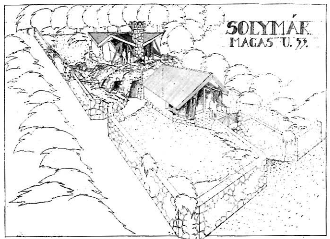
Solymár, családi ház terve (1991)
