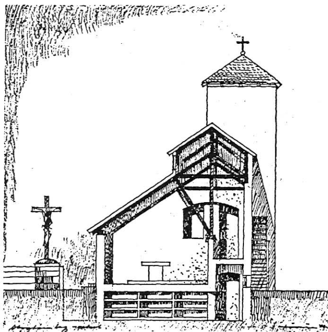
Ábrahámhegy, római katolikus templom metszete
