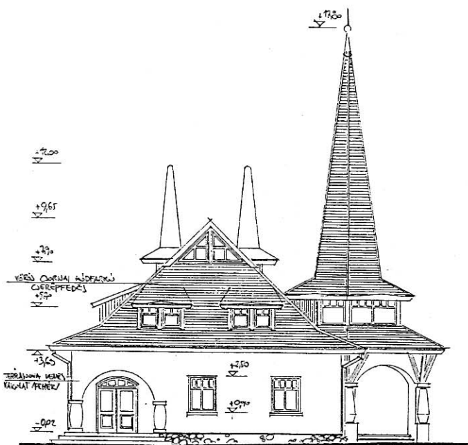
A 7.sz. (26. old.) adminisztrációs épület (Zsigmond László) és a 2.sz. oktatási épület (Bata Tibor) homlokzata
