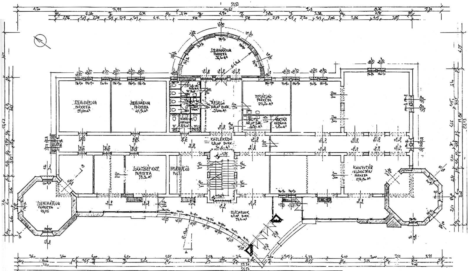
9.sz. (23. old.) és a 6.sz. (25. old.) oktatási épület átalakítási alaprajza és bejárati homlokzata (Siklósi József)
