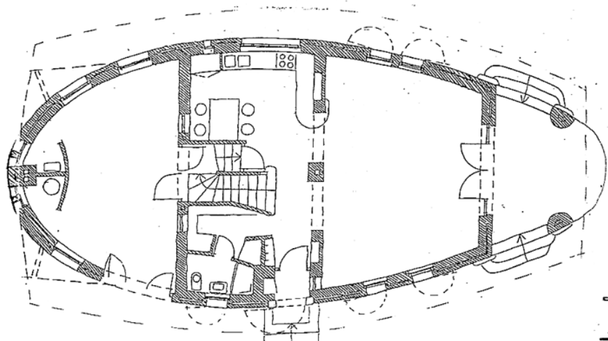
Családi ház a Duna-parton, Budakalász, 1993.
