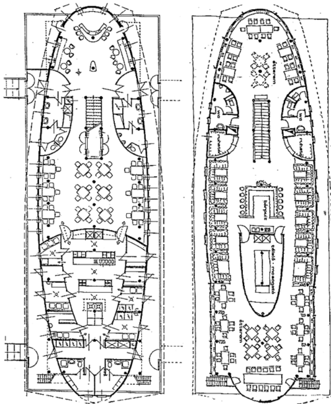
Étteremhajó a Volgán, Ribinszk, 1993. (Szerkesztő: Patyi György)
