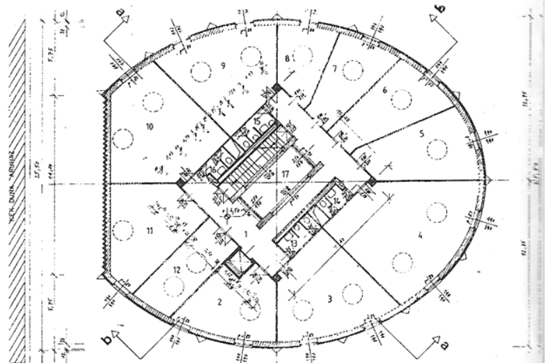
Dunaújváros, üzletház tervei, 1994.
