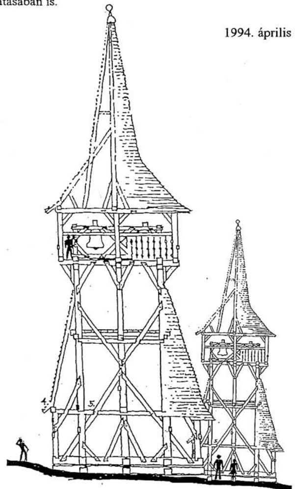
Szerkezeti nézetrajz, a nagyított (1,8:1) és az eredeti (1:1) méret összehasonlításával M = 1:100
