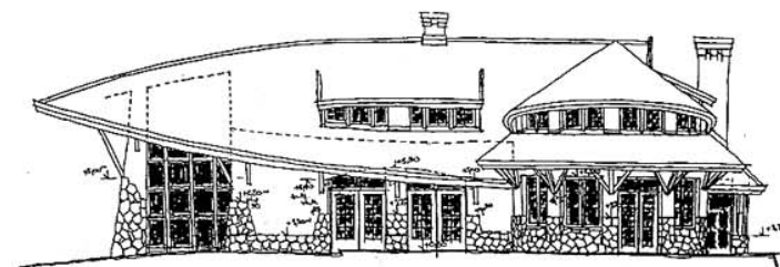
Kőműves-ház, Budakalász-Duna-part, 1993. (Szerkesztő Kővér István)
