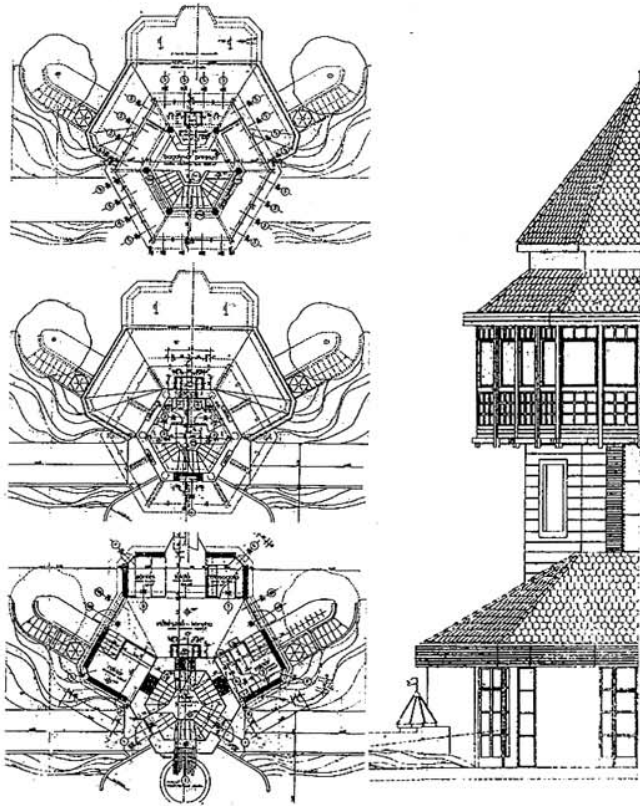
Kecskemét, Vízmű-térség, egykori katonai lőportorony (víztorony) hasznosítási terve, 1988
