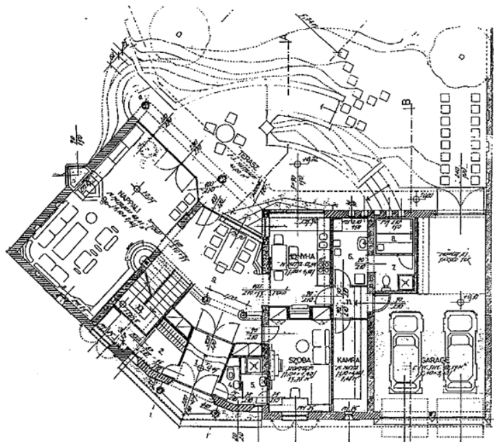
Kecskemét, Dr. Nemes-ház, 1992
