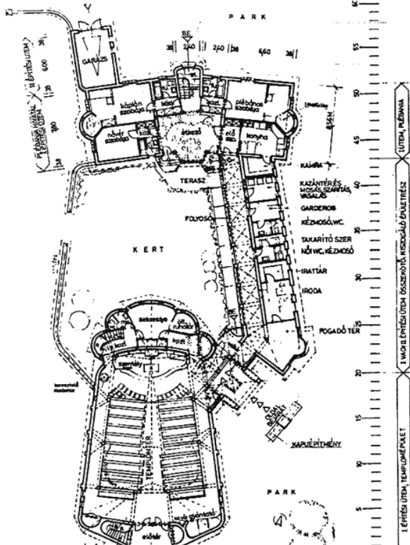
KATOLIKUS TEMPLOM – Békéscsaba
