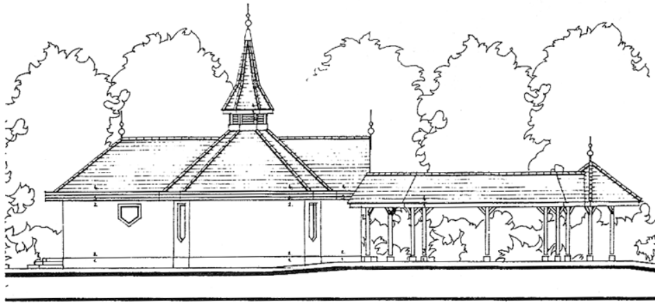
LAKÓHÁZ ÜZLETTEL – 1987 Tiszakécske (Az ácsmunkát egy segédmunkással magam készítettem)
