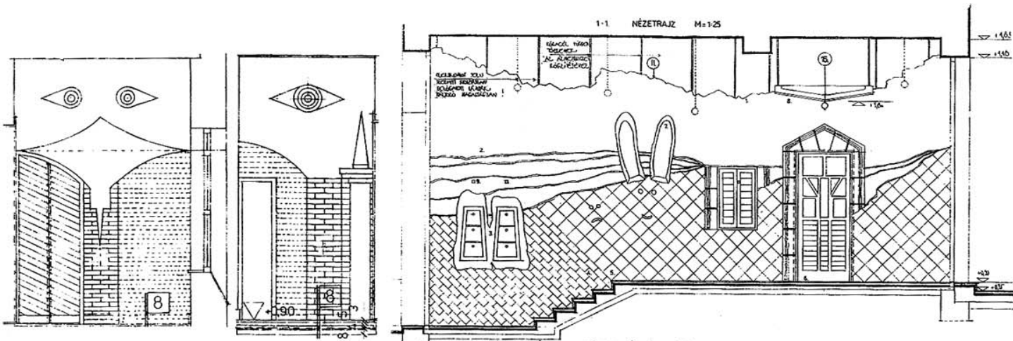
KŐHÍD UTCAI FOGHÍJ 1994 (Bozsódi – Pankotai)
