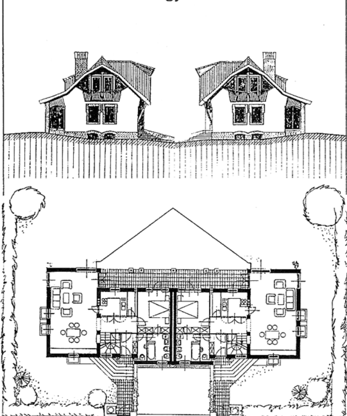
IKERHÁZ – Balassagyarmat
