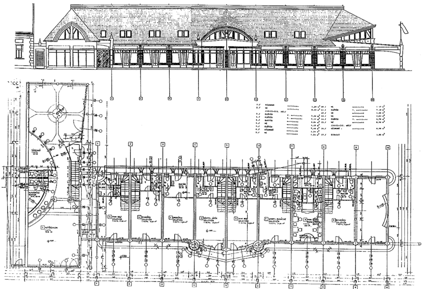
László, főtéri üzlet- és lakóház, 1994
