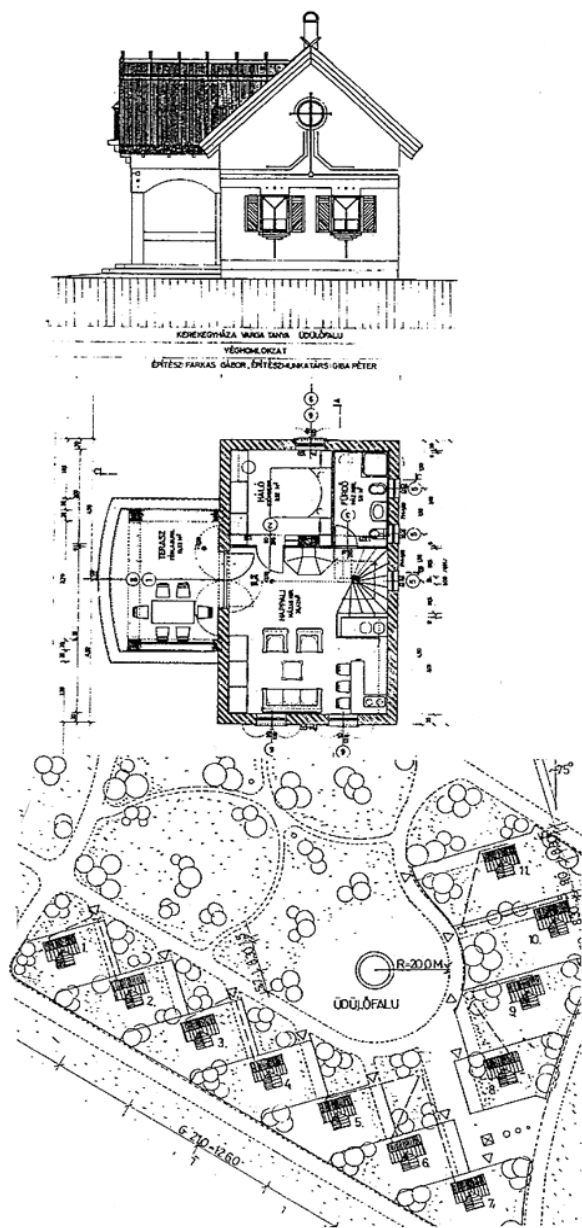
VARGA TANYA ÜDÜLŐFALU – Kerekegyháza (Farkas Gáborral)
