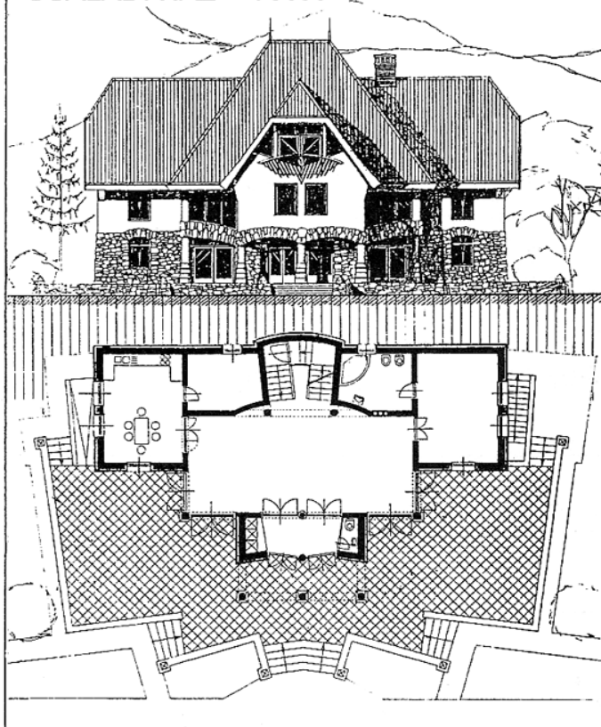
CSALÁDI HÁZ – Técső
