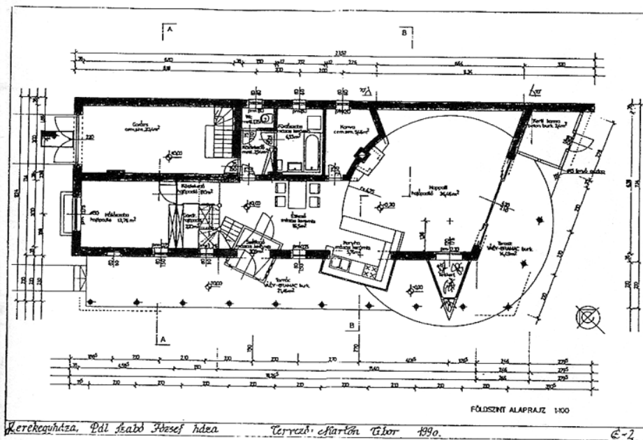
CSALÁDI HÁZ – Kerekegyháza
