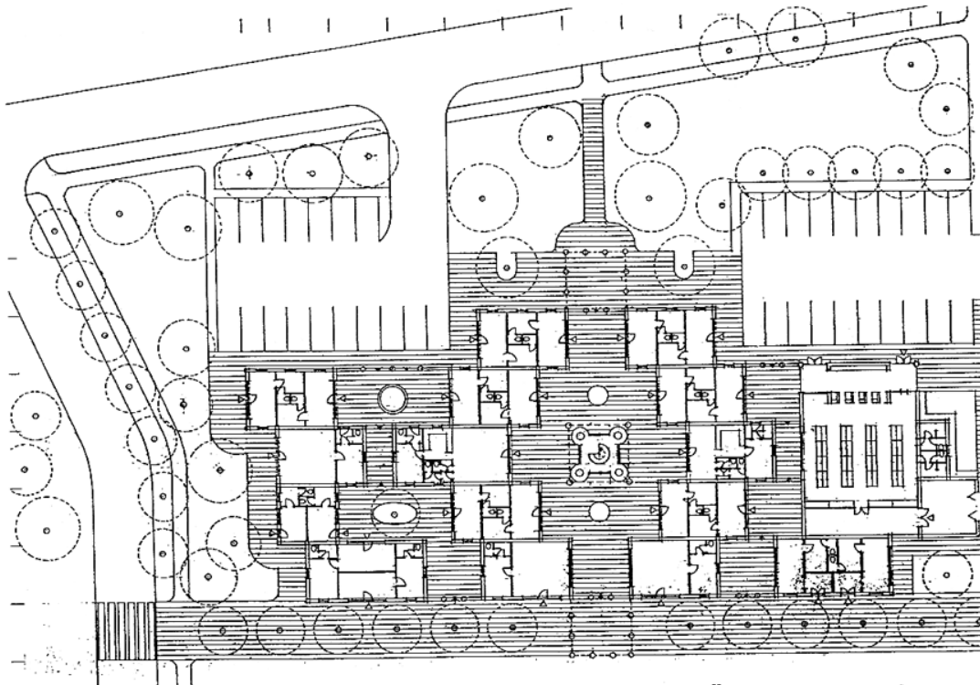
ÜDÜLŐFALU, ÜZLETEGYÜTTES – Nagybaracska
