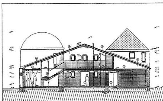
CUKRÁSZÜZEM – Kecskemét, 1994
