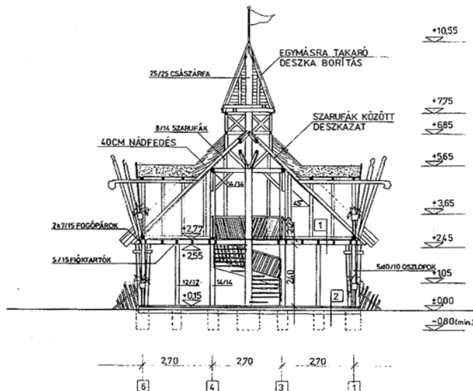
VENDÉGHÁZ ÉS FEDETT-NYITOTT SZÍN, 1994 – Lajosmizse – Ricsovári-major (Farkas Gáborral)
