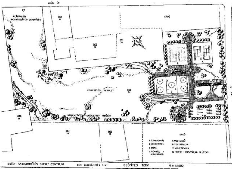
Nyír, szabadidő- és sportcentrum, beépítési terv, 1993 (Katkics Tamással)
