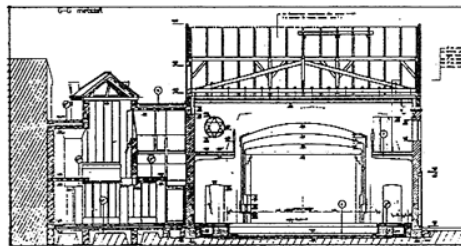
BÁBSZÍNHÁZ – Kecskemét, 1989 (2. változat, újabb változatként itt készült el a Magyar Fotográfiai Múzeum)
