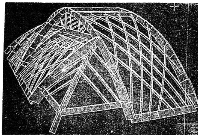
Az ívrács erőjátéka és a csarnok végének számítógépes modellje Az épület modelljét és a felvételeket Dankó István készítette
