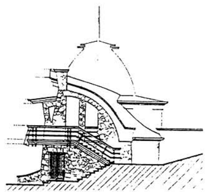
Piliscsaba, Katolikus Egyetem, teniszklub és fedett uszoda – Robogány Andrea diplomaterve (BME Középülettervezési Tanszék). Fent: a klubház távlati képe (Anthony Gall), nyugati és déli homlokzata; lent: az úszócsamok metszetei, véghomlokzata és a tető felülnézetének részlete.
