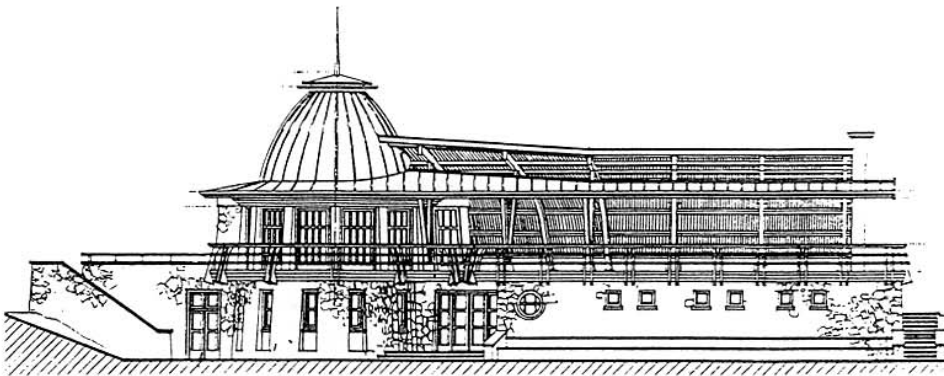
Piliscsaba, Katolikus Egyetem, teniszklub és fedett uszoda – Robogány Andrea diplomaterve (BME Középülettervezési Tanszék). Fent: a klubház távlati képe (Anthony Gall), nyugati és déli homlokzata; lent: az úszócsamok metszetei, véghomlokzata és a tető felülnézetének részlete.
