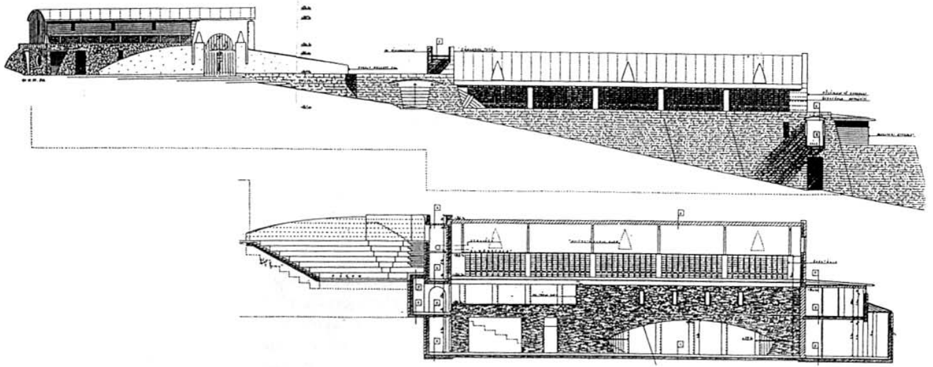
Tomaterem és töbrcélű csamok kiviteli terve. Az előző oldalon: hosszmetset és alaprajzok; jobbra fent: északi homlokzat, hosszmetset, keresztmetset és nyugati homlokzat.
