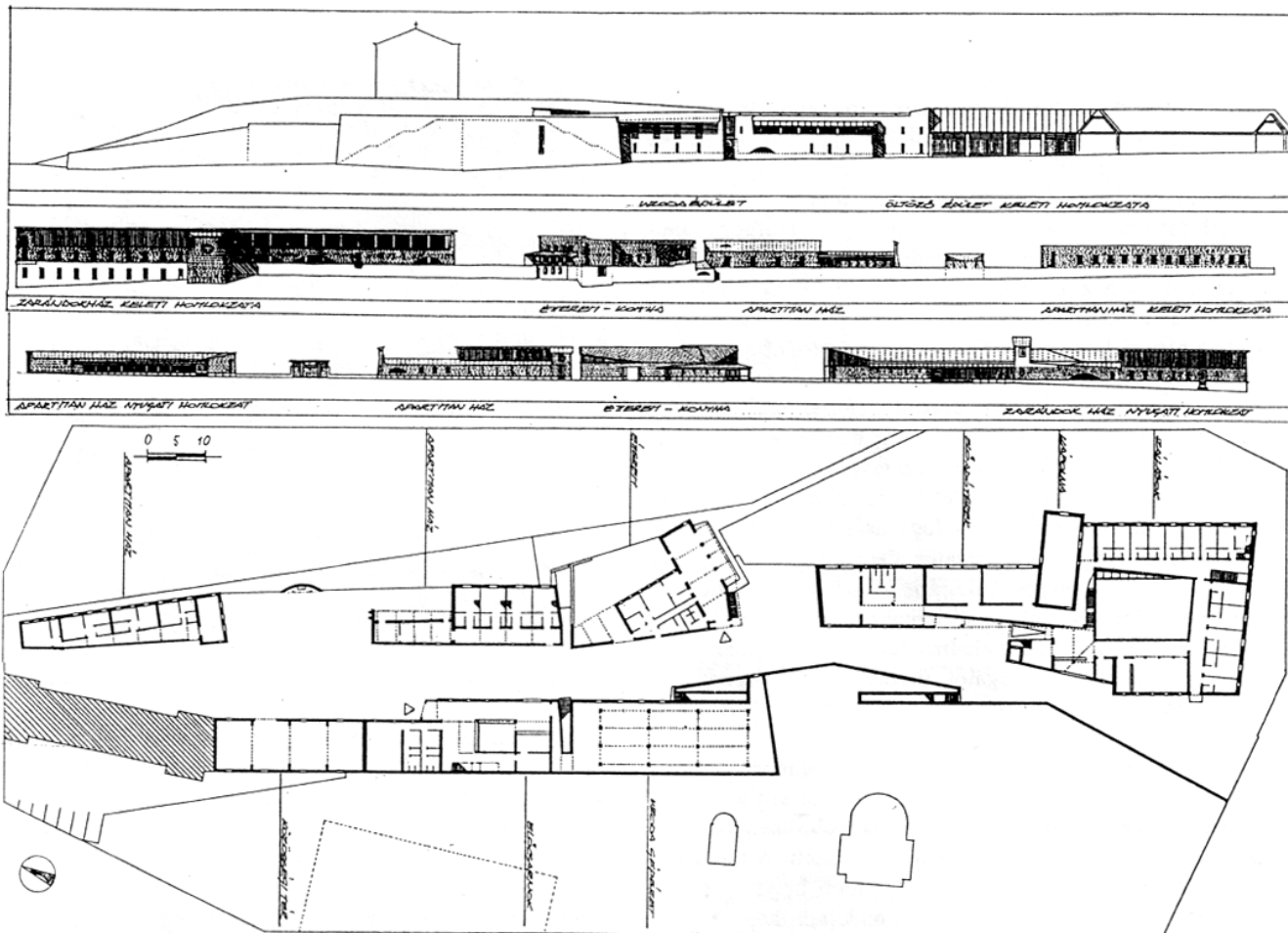
Lelkiségi központ alaprajza és homlokzatai – tanulmányterv
