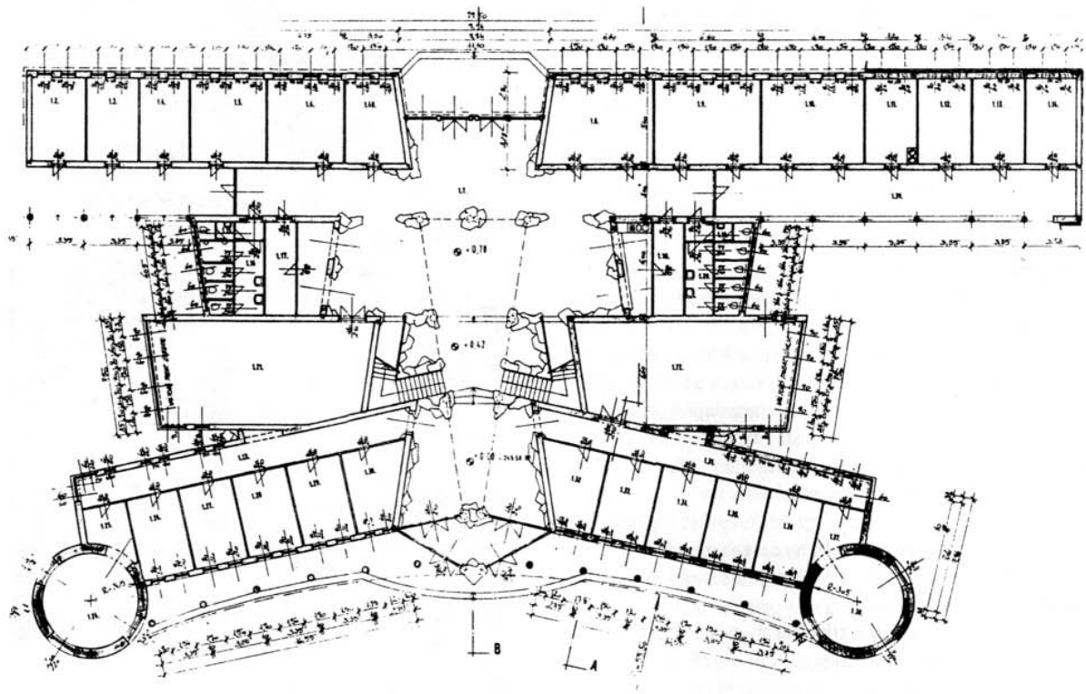
Az új oktatási épület, az Ambrosianum terve; alaprajz, homlokzat és keresztmetszet az épület tengelyében – építész: Siklósi József
