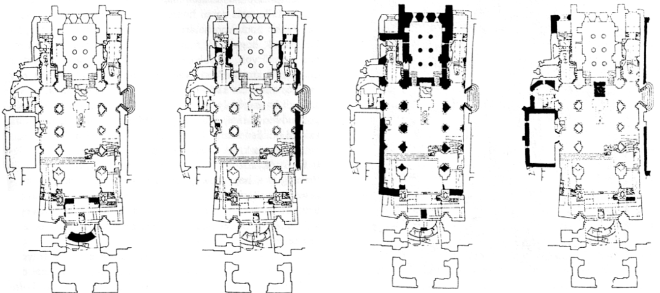
A bazilika összesítő ásatási alaprajza és hosszmetSZete, lent feketével jelölve a feltárt, XI. századi apszis, a XII. századi templomfalak, a XIII. századi falak és pillérek, valamint a XV. század végi kápolna és sekrestye. A kerengő falán lévő freskót az utolsó rajzon jobboldalt látható falmegerősítés takarja. (Rajz: László Csaba és Koppány Tiborné; a Műemlékvédelmi Szemle 1995/1-2 számából)
