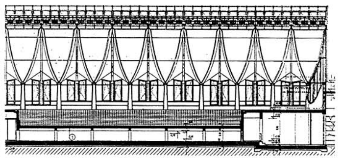
Piliscsaba, Katolikus Egyetem, teniszklub és fedett uszoda – Robogány Andrea diplomaterve (BME Középülettervezési Tanszék). Fent: a klubház távlati képe (Anthony Gall), nyugati és déli homlokzata; lent: az úszócsamok metszetei, véghomlokzata és a tető felülnézetének részlete.
