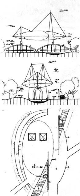
Szeged, többfunkciós tér. A kapuval és tomyokkal a Dóm teret jelképező „Tisza-híddal” és földsáncal határolt, fedett téren előadások, gyűlések és kiállítások rendezhetők.
