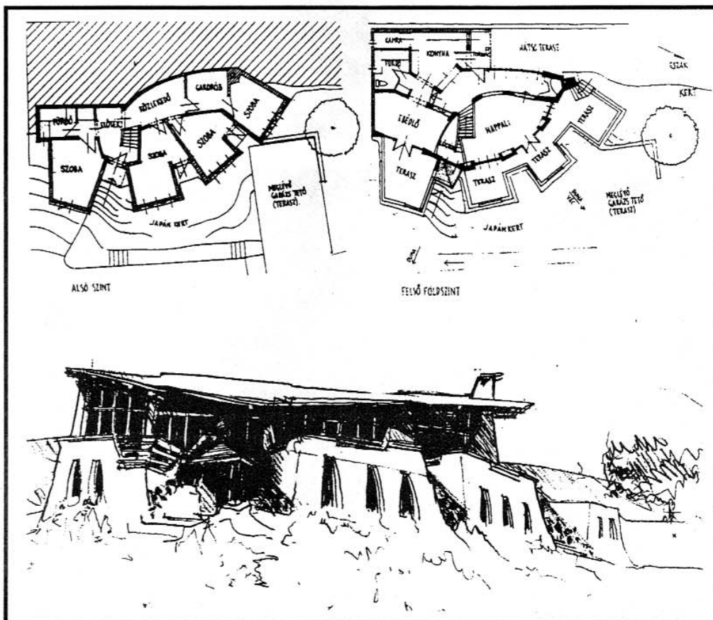
Tengőd, műemlékjellegű parasztház helyreállítási és bővítési terve, 1995
