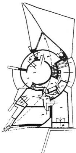
Martonvásár, Takács-ház, 1992 távlati kép és alaprajzok
