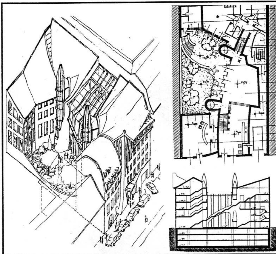
Budapest, VIII. Gyulai Pál utca irodaház 1993, (Róth Renátával és Engelmann Tamással)
