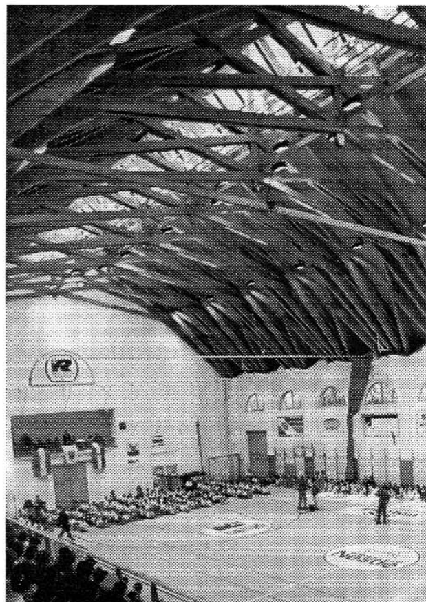
A szerencsei iskola tornaterme (Tusnady Zsolt felvétele)
