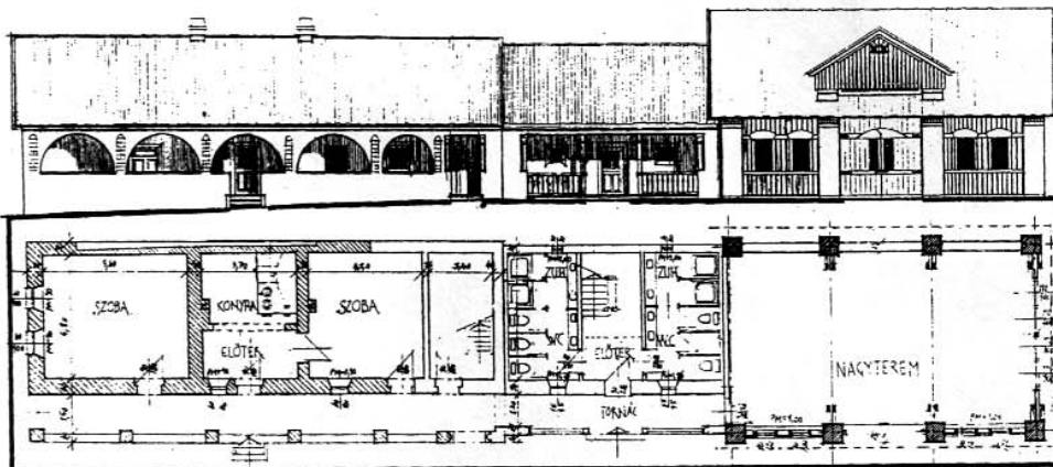
Tengőd, műemlékjellegű parasztház helyreállítási és bővítési terve, 1995
