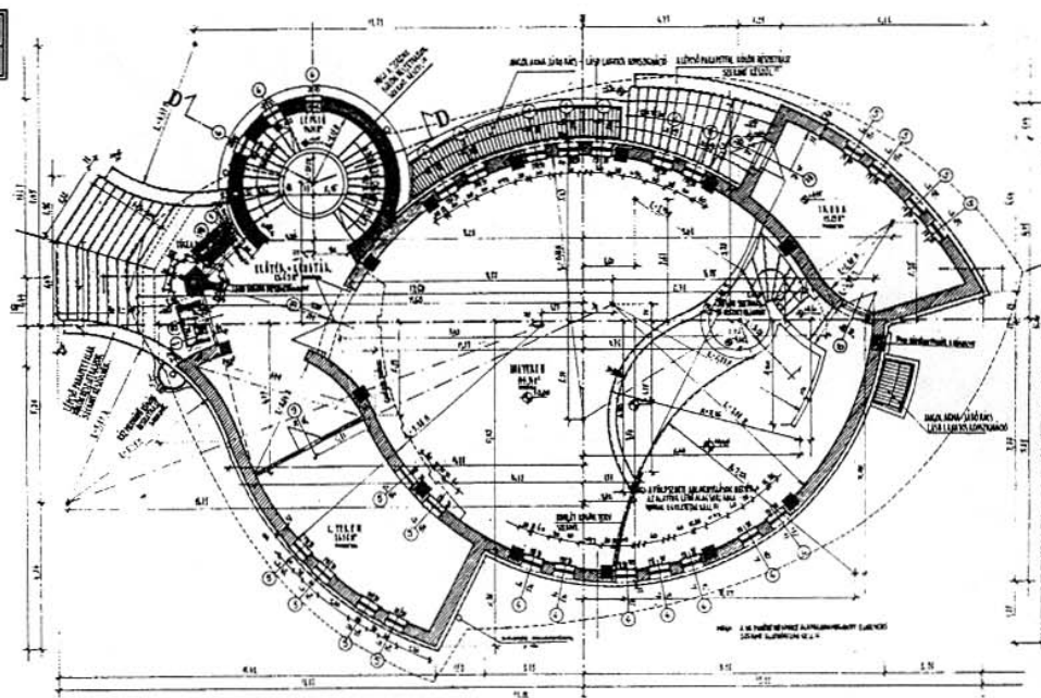
Veregyház, baptista templom, 1995, alaprajzok, metszetek, homlokzatok
