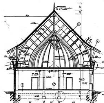
Csenger, polgármesteri hivatal, 1993-94, alaprajz, főhomlokzat, metszetek, modellfotó és a kész épület
