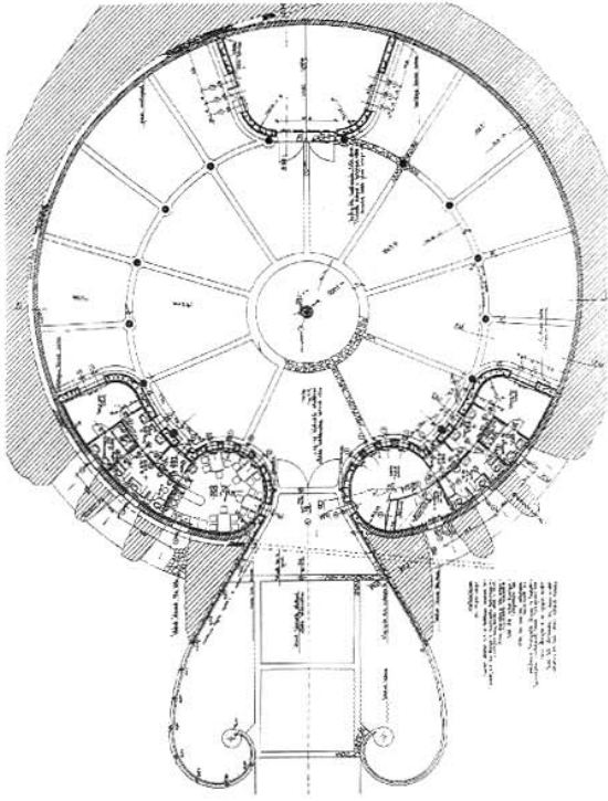
Borászok épülete a borfeldokozó felől és udvara (fotó: Ekler) (alsó képek) és alaprajza
