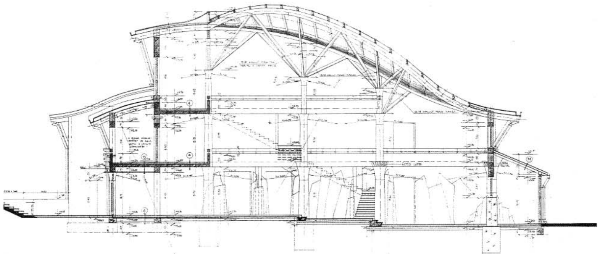
Piliscsaba, katolikus egyetem, épülő oktatási épület (Ambrosianum) metszete 1996, Siklósi József
