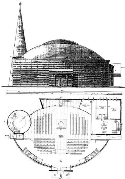
Református templom BME diplomaterv 1995 Halmai Attila (konzulens Balázs Mihály) diplomadíj, Lakóterv különdíj, északi homlokzat és alaprajz
