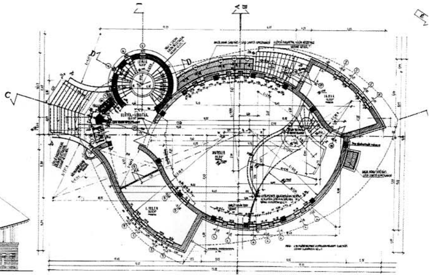
Veresegyház, Baptista templom főhomlokzata és alaprajza Zsigmond Ágnes, 1995
