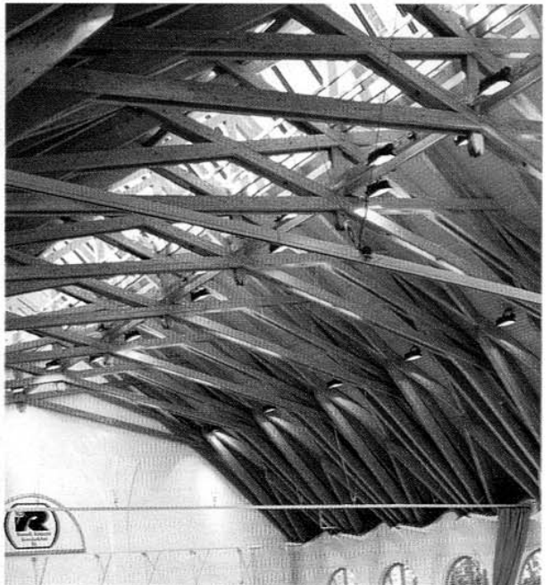
Szerencs, Bolyai iskola és sportcsarnok: udvar, és a csarnok tetőszerkezetének részlete (fotó: Tusnády)
