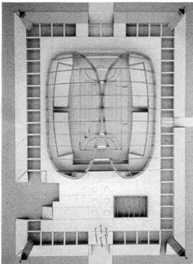
Tiszaújváros, sportcsarnok, pályaterv, Bodonyi Csaba 1996, homlokzat, metszet és modellfotók
