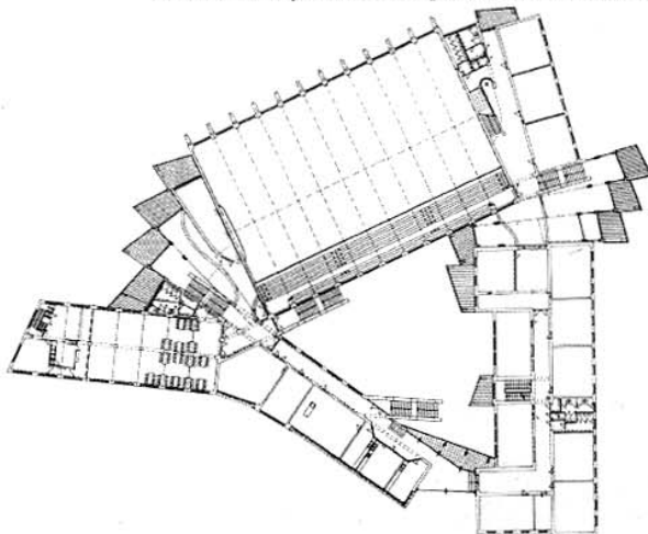
Szerencs, Bólyai iskola és sportcsarnok emeleti alaprajz és Posta utcai homlokzat, Salamin Ferenc 1989-96
