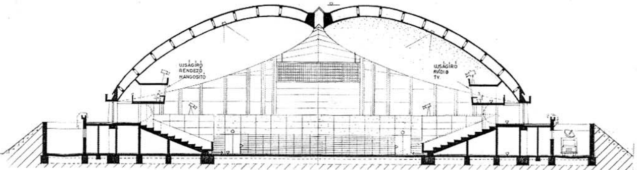
Tiszaújváros, sportcsarnok, pályaterv, Bodonyi Csaba 1996, homlokzat, metszet és modellfotók
