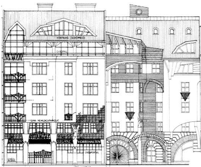
Budapest, IX. Angyal utca 33. lakóház, Kravár Ágnes, 1995 (a mellette lévő ház Dévényi Sándor terve) utcai homlokzatok
