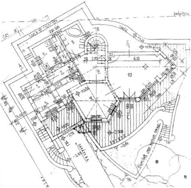
Budaörs, családi ház alaprajza és homlokzata, Kravár Ágnes
