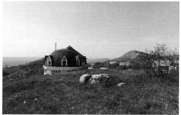
Budaörs, Nap-hegy, családi ház, Sáros László, munkatárs: Borzsák Lilla, 1991-93 Budaörs, Fodros utca, családi ház Sáros László, munkatárs: ifj. Lőrincz Ferenc, 1995-96
