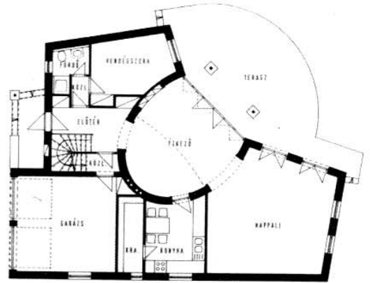
Solymár, családi ház földszinti és tetőtéri alaprajz, 1992-1993 Tusnády Zsolt
