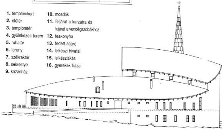
Dunaujváros, evangélikus templom alaprajza és oldalhomlokzata Nagy Tamás
