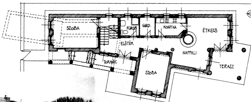
Vándoriskolás diplomamunka: Máriahalom, Lakatos-ház – utcai és udvari homlokzat és földszinti alaprajz
