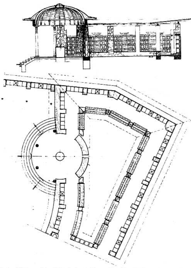
Szabadtéri ravatalozó és kolumbárium alaprajza és keresztmetszete
