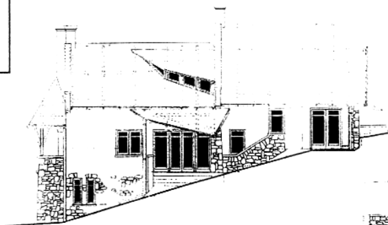
Pilisjászfalu, Reisz-ház kiviteli terve, 1996 – alaprajzok, homlokzatok és távlati kép
