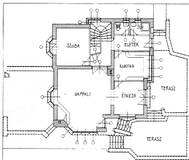
Pilisjászfalu, Gerő-ház kiviteli terve, 1996 – alaprajzok és távlati kép
