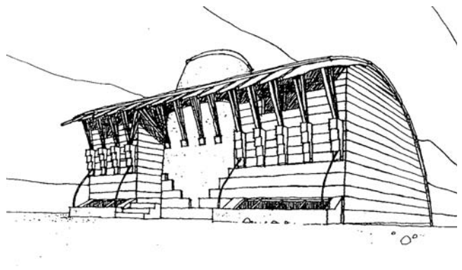
Kovács Imre nyaralóháza Szigetszentmiklós, 1994-95; munkatársak: Páricsy Zoltán, Pintér Balázs Távlati képek, hossz- és keresztmetszet, földszinti és tetőtéri alaprajz.
