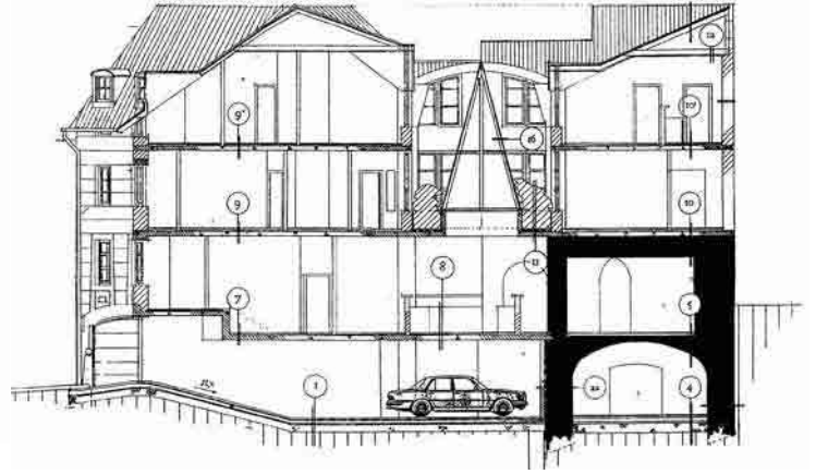
Iroda- és lakóépület , Budapest, Szalag utca, 19., 1996-98, munkatársak: Páricsy Zoltán, Szólik Krisztina, Jakab Csaba, Gulybán Ede, Révai Attila. A ház alatt középkori falmaradványok találhatóak, amelyek feltárását követően termv módosításra volt szükség, hogy bemutathatók legyenek. Távlati kép, keresztmetszet, pince, földszint, emelet és tetőtér alaprajza.
