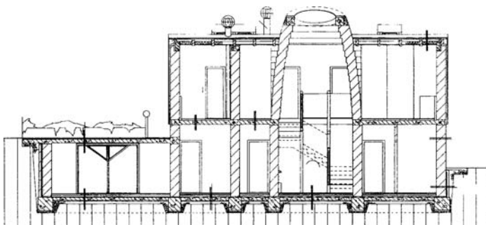
Kovács Imre nyaralóháza Szigetszentmiklós, 1994-95; munkatársak: Páricsy Zoltán, Pintér Balázs Távlati képek, hossz- és keresztmetszet, földszinti és tetőtéri alaprajz.
