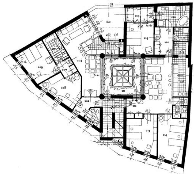
Iroda- és lakóépület , Budapest, Szalag utca, 19., 1996-98, munkatársak: Páricsy Zoltán, Szólik Krisztina, Jakab Csaba, Gulybán Ede, Révai Attila. A ház alatt középkori falmaradványok találhatóak, amelyek feltárását követően termv módosításra volt szükség, hogy bemutathatók legyenek. Távlati kép, keresztmetszet, pince, földszint, emelet és tetőtér alaprajza.
