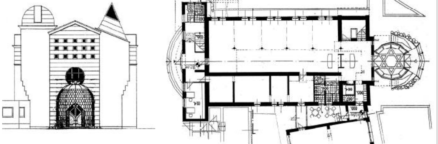
A tervezett jászberényi könyvtár kereszt- és hosszmet-szete, főhomlokzata, földszinti és emeleti alaprajza
