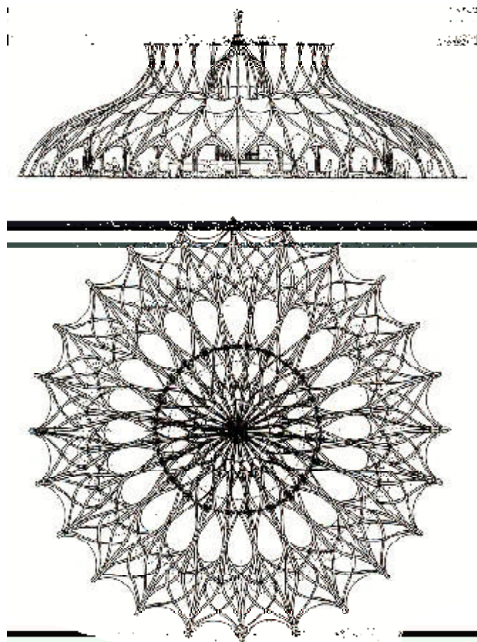
Marcel Kalberer és munkatársai élő építményeinek két példája. Fent: az Auerworld Palace, Auerstedt, 1998; alaprajz és homlokzat. Lent: Victoria-pavilon, Malmö, 2001; alaprajz és a szerkezet távlati képe
