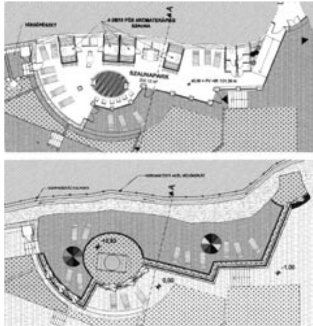
Fent: a szaunapark alaprajzai; lent: a 60-as években elbontott tavi fürdő rekonstrukciója
