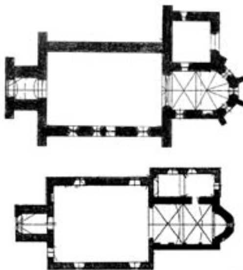
A bántornyai és a mártonhelyi középkori templomok alaprajza
